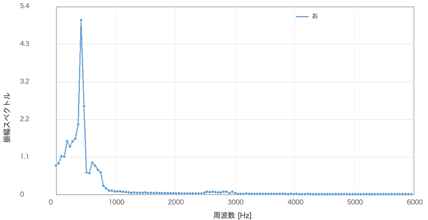
図 11: 母音「お」の振幅スペクトル
