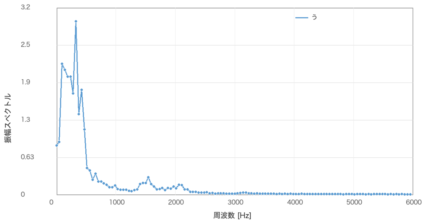
図 9: 母音「う」の振幅スペクトル
