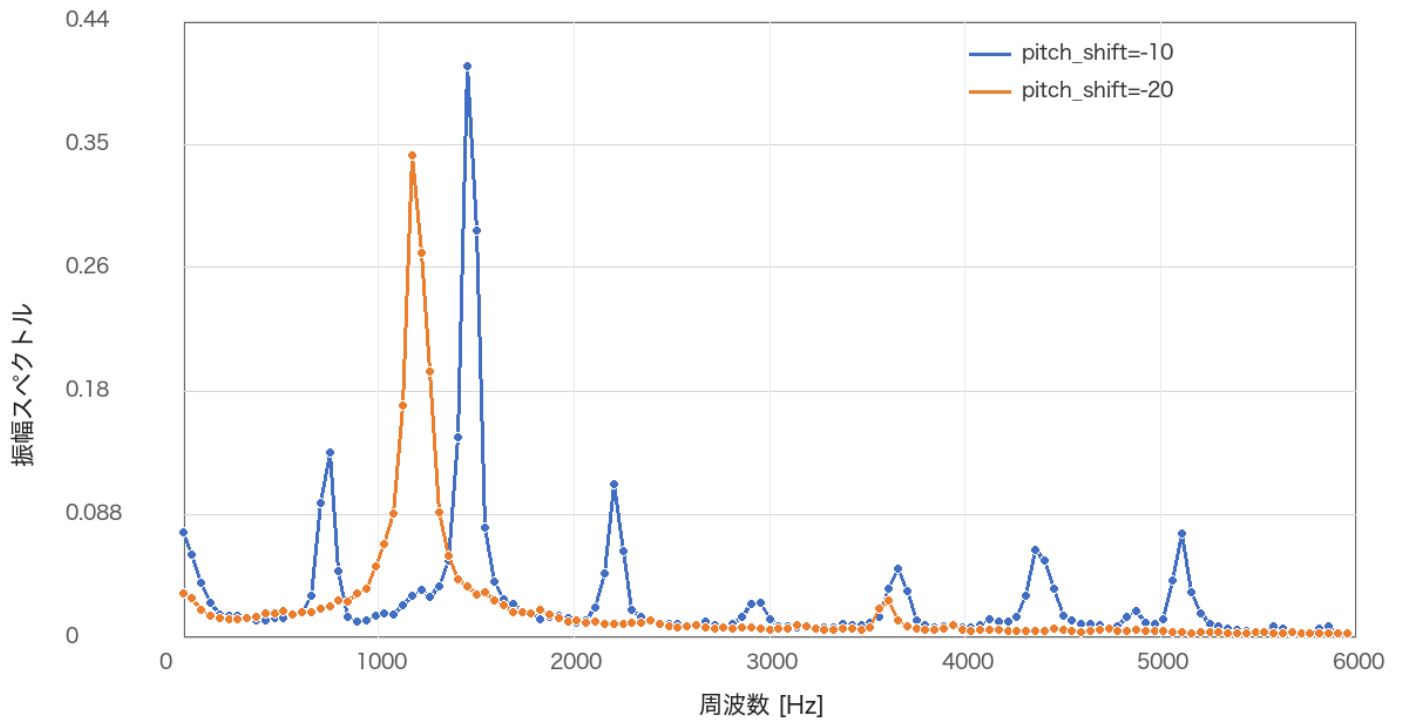
図 6: pitch_shift の設定値による振幅スペクトルの比較
