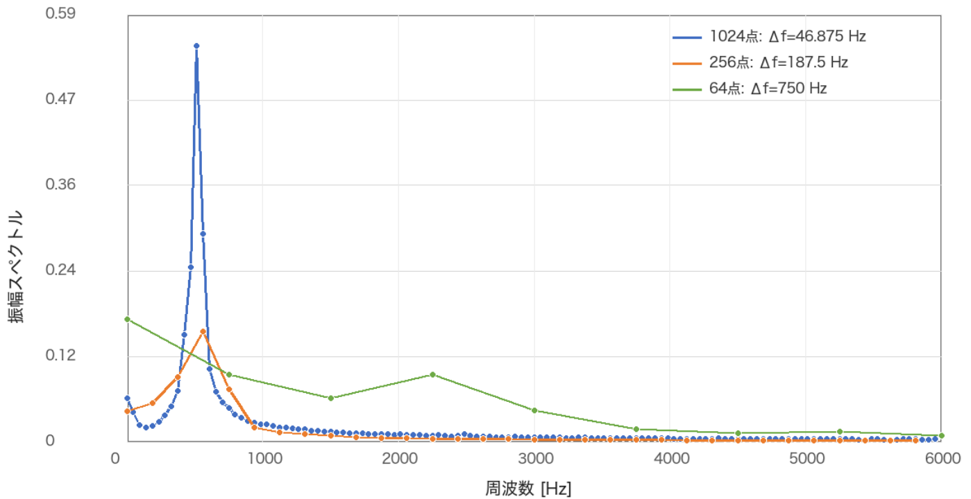
図 5: サンプル数による振幅スペクトルの比較
