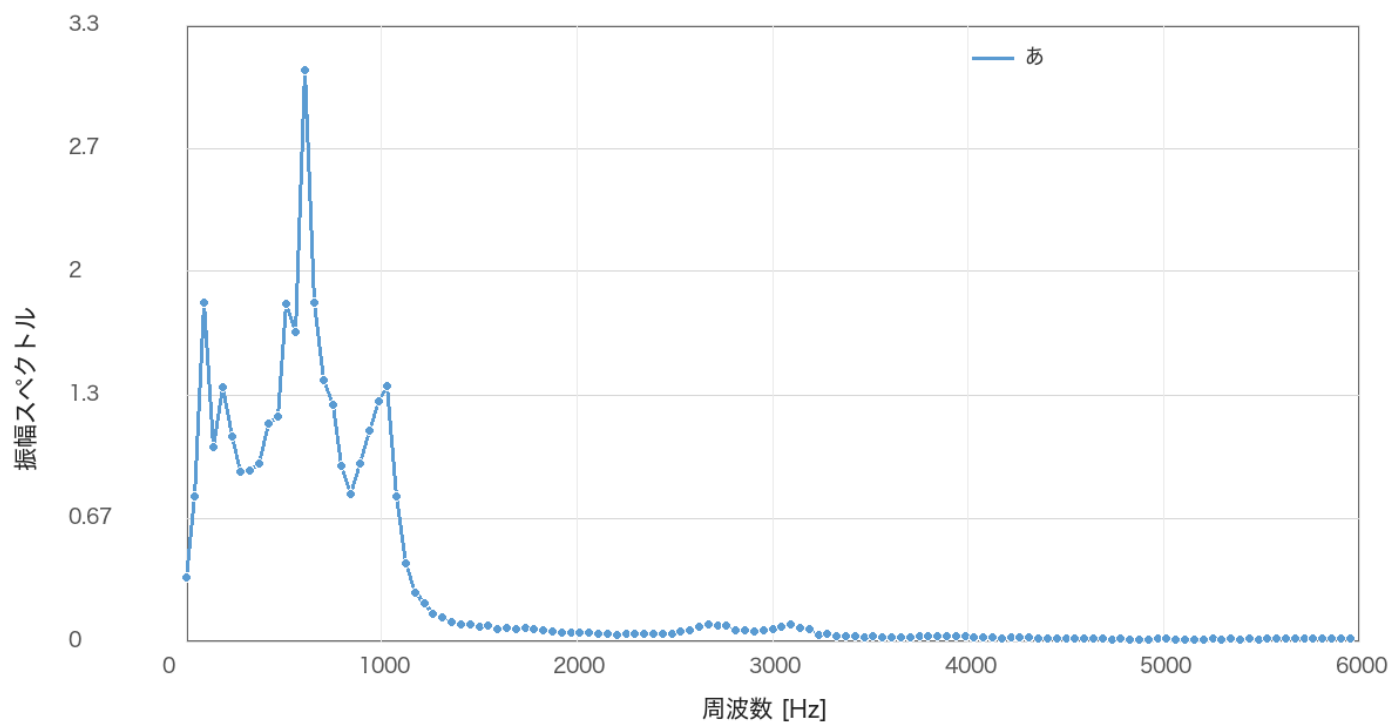
図 7: 母音「あ」の振幅スペクトル
