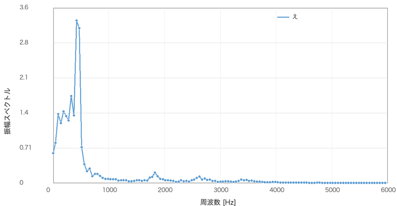
図 10: 母音「え」の振幅スペクトル
